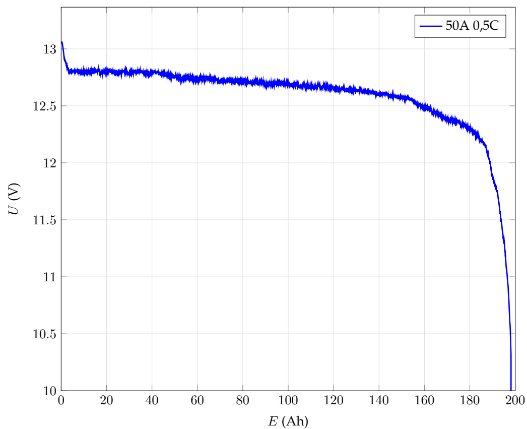
Vybíjení baterie WB4S-CH-200 proudem 50A
